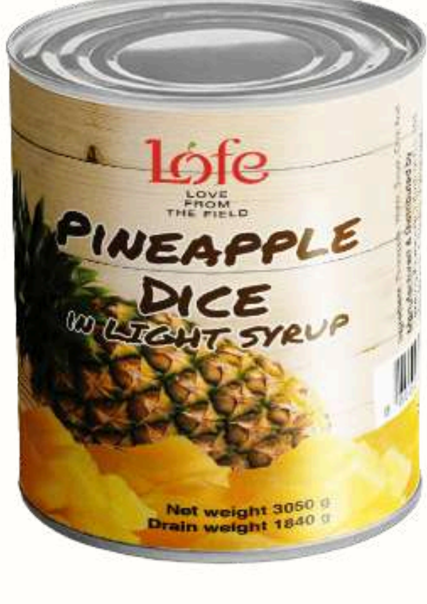
Dice
